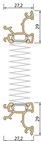
Zijgeleidingsprofiel
