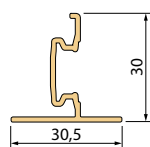
Verduisteringsprofiel
